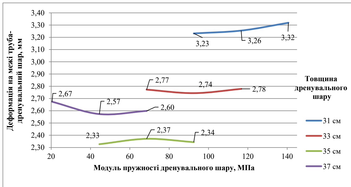
Рисунок 3 – Залежність деформацій Z від модуля пружності піщаного дренажного шару з полівінілхлоридною трубою
