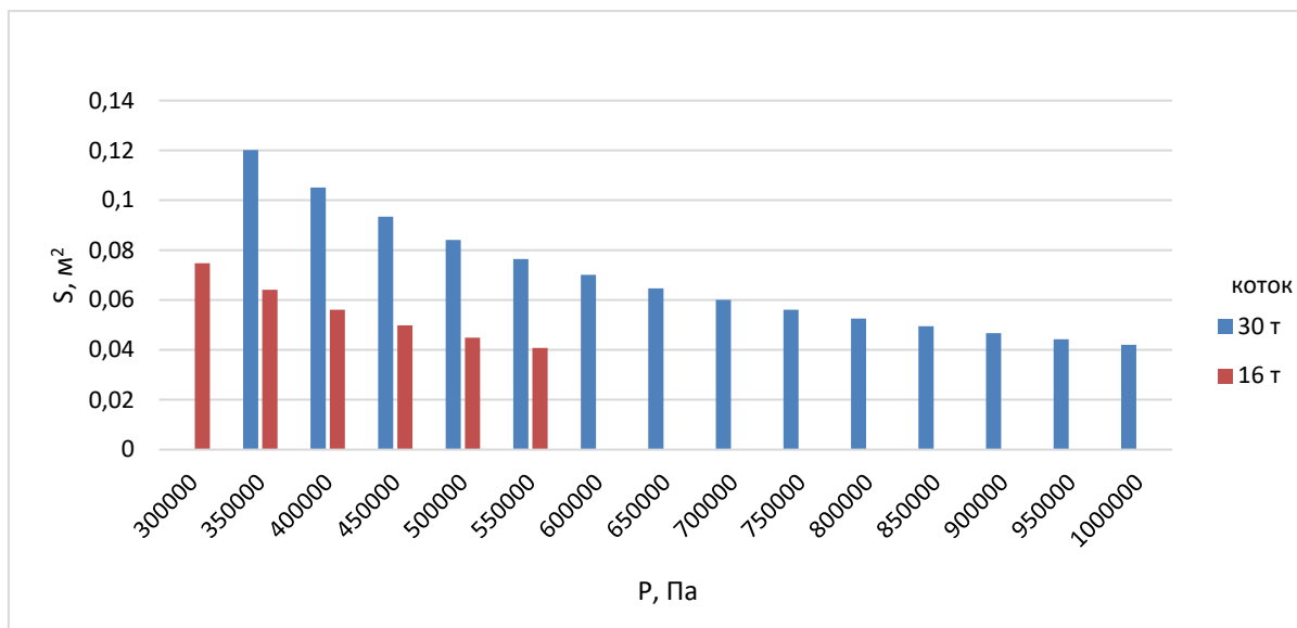
Рисунок 1 – Залежність площі штамбу котка від тиску в його шинах Figure 1 – Dependence of the area of the roller stamp on the pressure in its tires
