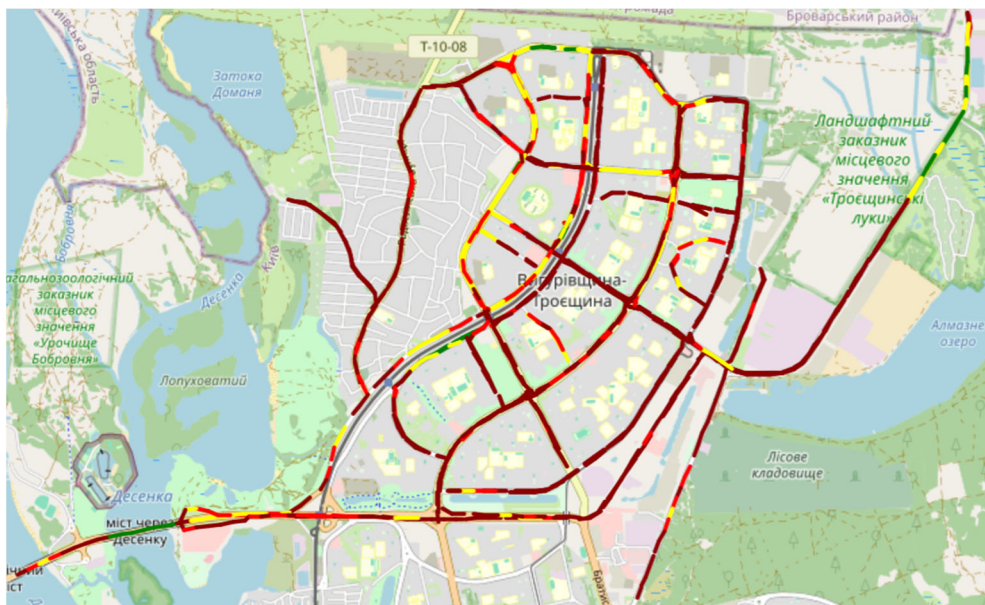
Рисунок 3 – Картограма районної вулично-дорожньої мережі за показником IRI
