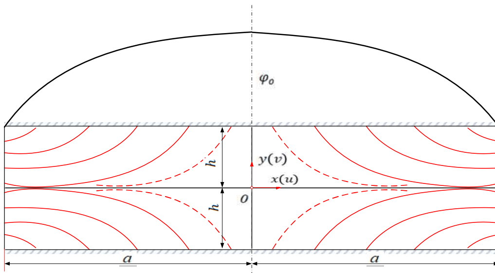
Рисунок 2 – Схема для розрахунку віддавлення пластичного ґрунту (за А. Надаї).
