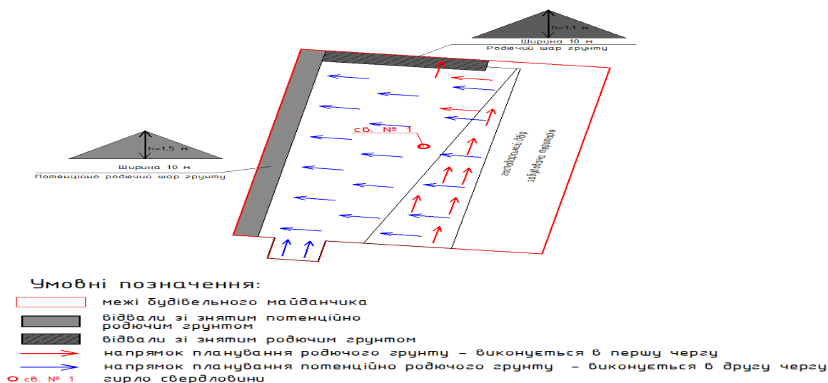
Рисунок 2 – Технологічна схема зняття родючого та потенційно родючого шарів ґрунту Figure 2 – Technological scheme for removing fertile and potentially fertile soil layers
