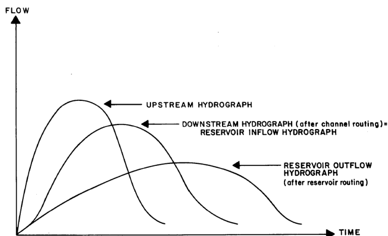
Рисунок 6 – Схема модифікації форми повеневого гідрографу
