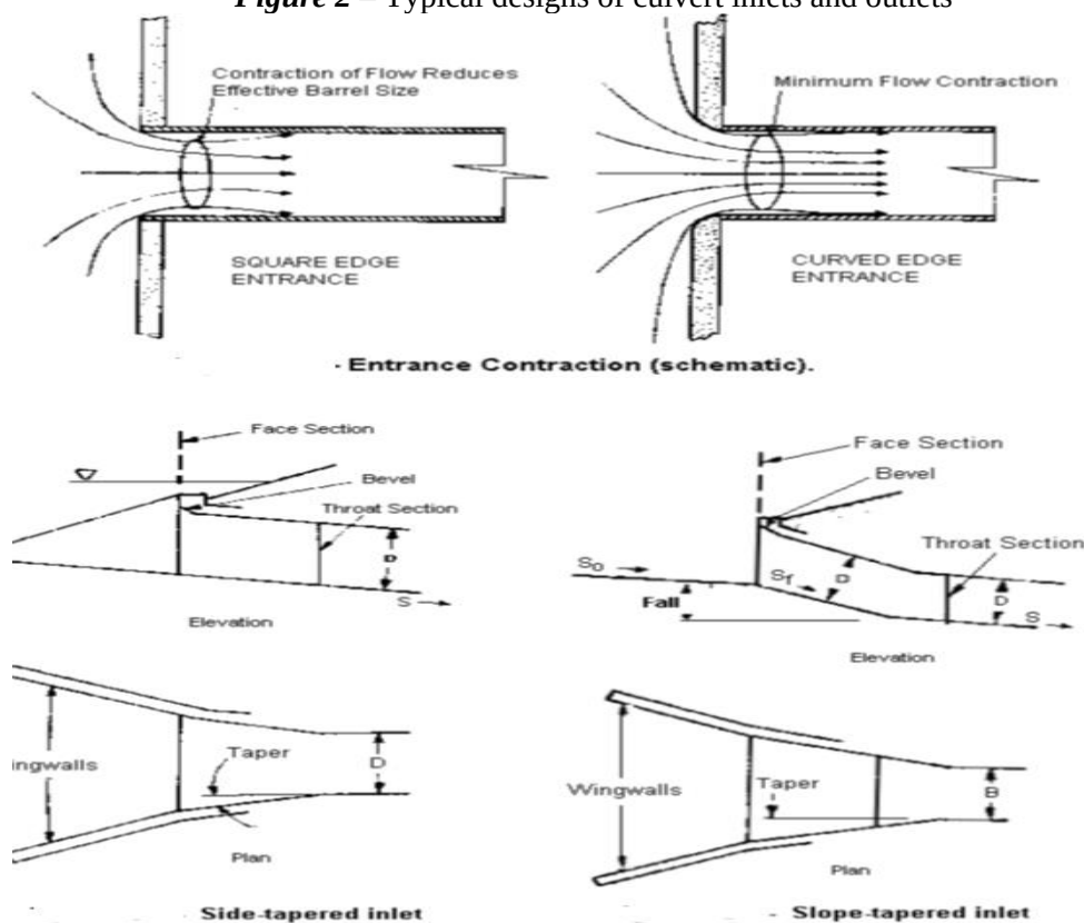
Рисунок 2 – Типові конструкції входних та вихідних отворів ВП Figure 2 – Typical designs of culvert inlets and outlets
