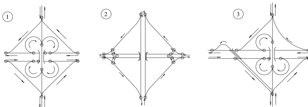
Рисунок 1 – Конфліктні точки на транспортних розв'язках
