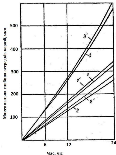
Рисунок 2. - Максимальна глибина осередків корозії. 1 - без добавки; 2 - добавка ТНХК; 3 - добавка CaCl 2 при нормальному твердінні; 1', 2', 3' - ті ж, після тепловологої обробки
