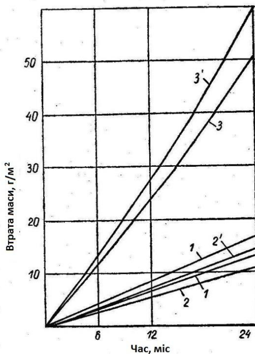
Рисунок 1. - Кінетика втрати маси сталевих арматурних стержнів 1 - без добавки; 2 - добавка ТНХК; 3 - добавка \text{CaCl}_2 при нормальному твердінні; 1', 2', 3' - ті ж, після теплової обробки
