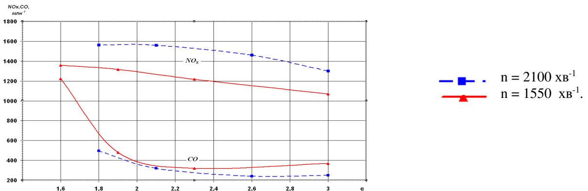
Рисунок 4 – Токсична характеристика ВГ дизеля СМД при n = 2100 і 1550 \text{ хв}^{-1}
