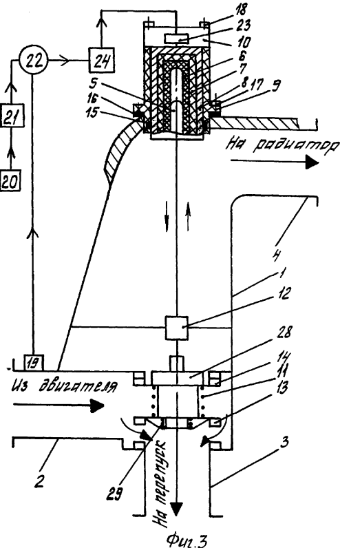
Рисунок 6 – Термостат [8].
