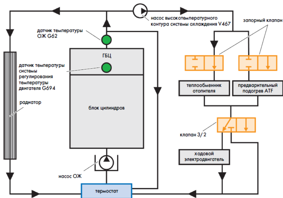
Рисунок 4 – Схема (приклад) [7].
