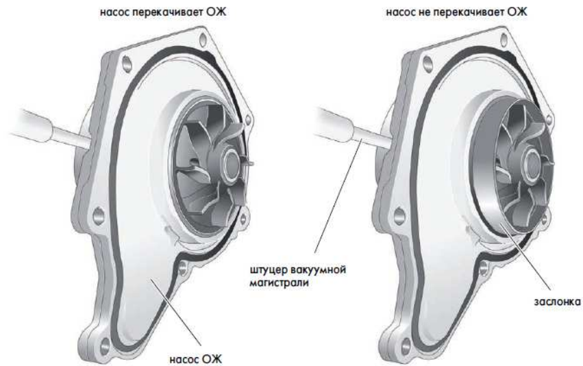
Рисунок 5 – Насос системы охлаждения [7].
