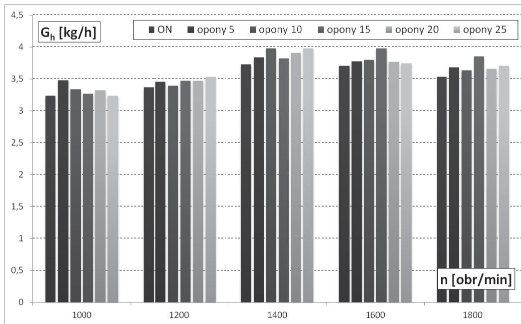
Rys. 4. Godzinowe zużycie paliwa silnika badawczego zasilanego badanymi paliwami
