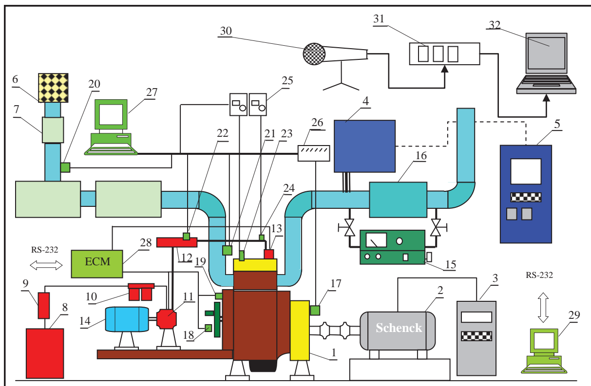
Rys. 2. Schemat stanowiska pomiarowego: 1 – silnik badawczy SB3.1/CR5, 2 – hamulec hydrauliczny, 3 – pulpit sterowniczy hamulca hydraulicznego, 4 – układ poboru próbek spalin systemu pomiaru emisji PM, 5 – pulpit sterowniczy systemu pomiaru emisji PM, 6 – filtr powietrza, 7 – przepływomierz powietrza ze zbiornikami kompensacyjnymi, 8 – system pomiaru zużycia paliwa, 9 – pompa zasilająca, 10 – zespół filtrów, 11 – pompa wysokiego ciśnienia CR, 12 – zasobnik ciśnienia CR, 13 – wtryskiwacz CR, 14 – silnik elektryczny napędzający pompę wysokiego ciśnienia, 15 – układ pomiaru zadymienia spalin, 16 – tłumik wydechu, 17 – czujnik indukcyjny pomiaru GMP, 18 – czujnik indukcyjny pomiaru położenia wału rozrządu, 19 – czujnik indukcyjny pomiaru prędkości obrotowej silnika, 20, 21 – czujniki ciśnienia bezwzględne 22 – czujnik ciśnienia w zasobniku CR, 23 – czujnik piezokrystaliczny ciśnienia w cylindrze, 24 – czujnik ciśnienia w przewodzie paliwowym łączącym zasobnik ciśnienia z wtryskiwaczem, 25 – wzmacniacze ładunku elektrycznego, 26 – kondycjoner sygnału, 27 – komputer rejestrujący szybkozmienne sygnały elektryczne, 28 – elektroniczny sterownik układu CR, 29 – komputer sterujący parametrami układu CR, 30 – mikrofon SF-21, 31 – NI CompactDAQ, 32 – laptop z oprogramowaniem LabVIEW z dodatkiem Sound and Vibration Toolkit [2]
