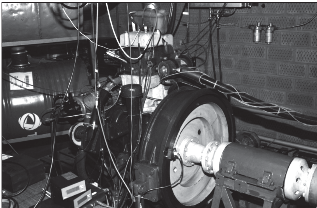
Rys. 1. Obiekt badań – jednocylindrowy silnik badawczy SB-3.1 z układem zasilania typu CR [2]
