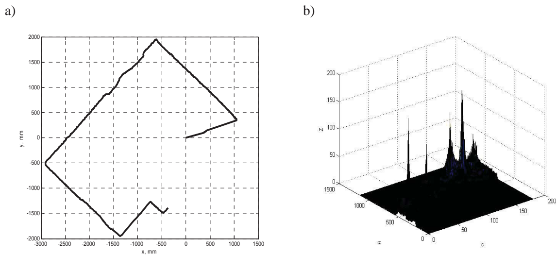
Rysunek 4. Zastosowanie transformaty Hougha: a) wyniki uzyskane na podstawie pomiarów dalmierza, b) wyniki stosowania transformaty Hougha przy obliczaniu odległości c i kąta \alpha
