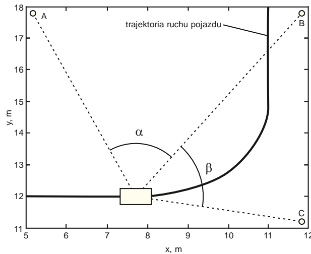
Rysunek 6. Przykładowy przebieg trajektorii pojazdu z zaznaczonymi znacznikami i kątami niamiaru
