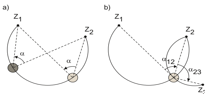
Rysunek 2. Ilustracja metody triangulacji: a) – dwa znaczniki: przypadek niejednoznaczny, b) – trzy znaczniki: rozwiązanie jednoznaczne.
