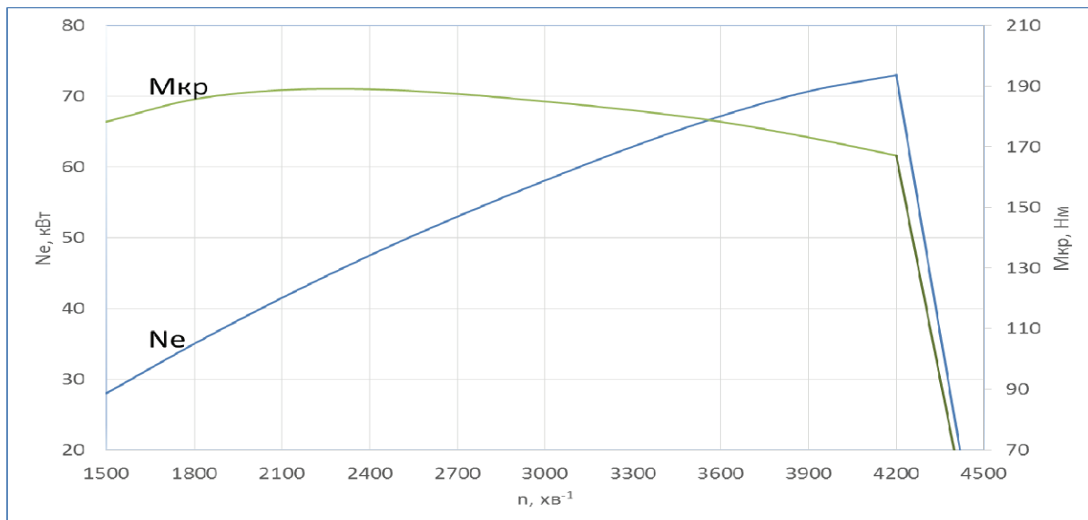
Рисунок 1 – Зовнішня характеристика дизеля 4ДТНА1
