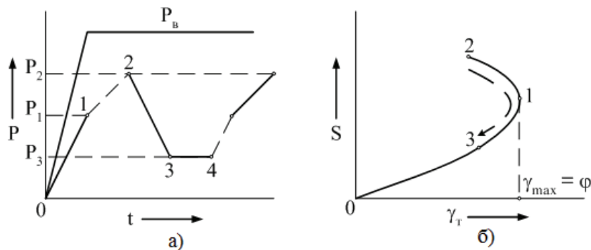
Рисунок 3 – Характеристики АБС
