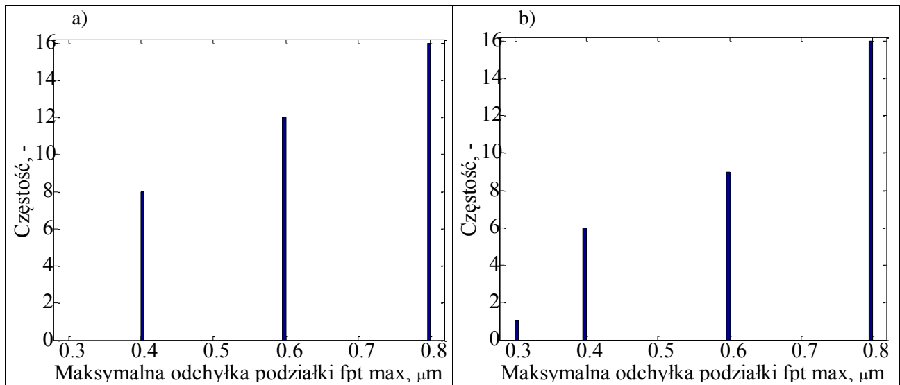
Rys. 5. Histogram wartości maksymalnej odchyłki podziałki f_{pt\ max} po: a) szlifowaniu (lewe boki 0,60 \pm 0,12, prawe boki 0,62 \pm 0,13), b) wygładzaniu (lewe boki 0,65 \pm 0,11, prawe boki 0,68 \pm 0,14) - w nawiasie wartość średnia i niepewność rozszerzona przy poziomie ufności 95%, \mu\text{m}
