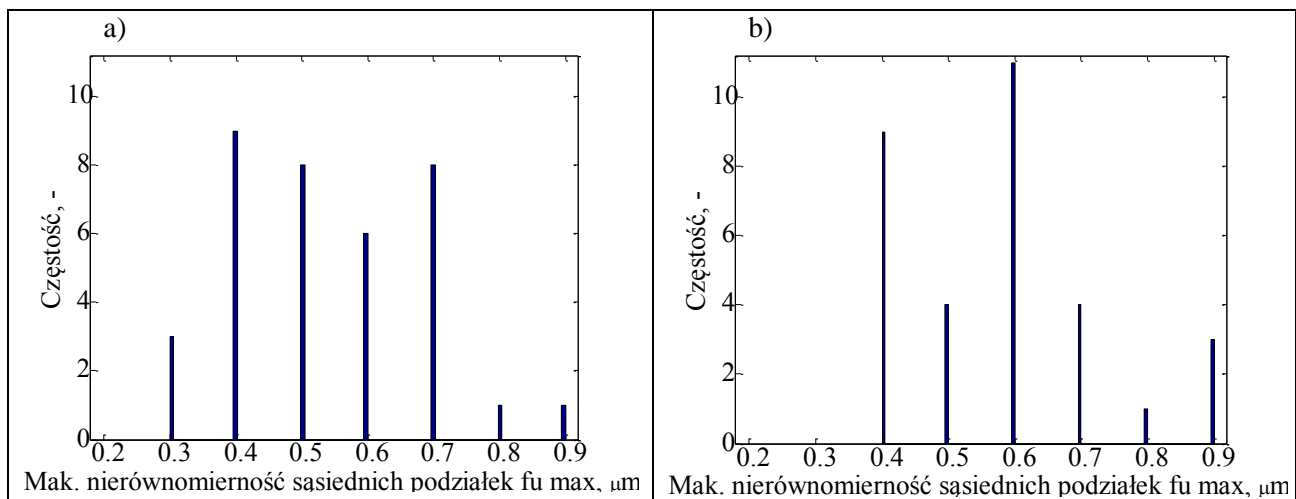
Rys. 6. Histogram wartości maksymalnej nierównomierności sąsiednich podziałek f_{u\ max} po: a) szlifowaniu (lewe boki 0,58 \pm 0,04, prawe boki 0,51 \pm 0,13), b) wygładzaniu (lewe boki 0,51 \pm 0,13, prawe boki 0,56 \pm 0,13) - w nawiasie wartość średnia i niepewność rozszerzona przy poziomie ufności 95%, \mu\text{m}
