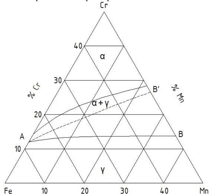
Рисунок 2 – Ізотермічний переріз при 1000 °С потрійної діаграми Fe–Cr–Mn (0,1% C)
