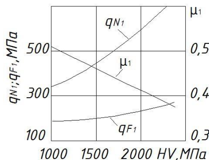
Рисунок 9 – Залежність контактних характеристик q_{N1} , q_{F1} та \mu_1 на задній поверхні інструмента (сталь Р18; \gamma = 15^\circ ; \alpha = 3^\circ ; h_3 = 0,1 мм) від твердості HV сталі 12X18H10T при вільному різанні ( v = 1,17 м/с; a_z = 0,1 мм; МОР — сульфифрезол)
