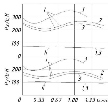
Рисунок 6 – Залежність складових сил різання P_z та P_y від швидкості v при вільному різанні сталі 12X18H10T різцем (сталь Р18; \gamma = 15^\circ ; \alpha = 3^\circ ; МОР — сульфохрезол) з товщиною зрізу a_z = 0,1 мм (I) та 0,03 мм (II) та шириною b : 1 – HV = 1080...1110 МПа; 2 – HV = 1840...1890 МПа; 3 – HV = 2220...2290 МПа
