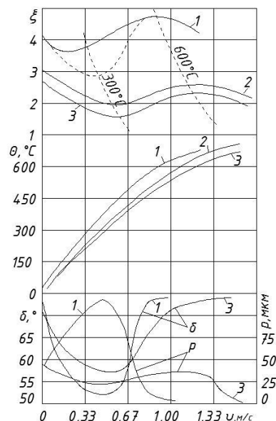
Рисунок 5 – Залежність усадки стружки \xi , температури різання \Theta , кута різання \delta та радіуса заокруглення \rho ріжучої кромки різця (сталь Р18; \gamma = 15^\circ ; \alpha = 3^\circ ; a_z = 0,1 мм; МОР — сульфохрезол) від швидкості різання при вільному різанні сталі 12X18H10T:
