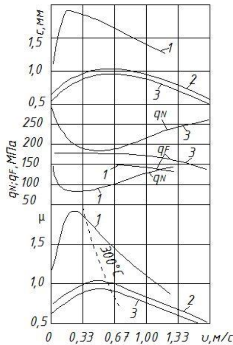
Рисунок 8 – Залежність контактних характеристик c , q_N , q_F та \mu від швидкості різання при вільному різанні сталі 12X18H10T різцем (сталь Р18; \gamma = 15^\circ ; \alpha = 3^\circ ; a_z = 0,1 мм; МОР — сульфифрезол): 1 – HV = 1080 \dots 1110 МПа; 2 – HV = 1840 \dots 1890 МПа; 3 – HV = 2220 \dots 2290 МПа
