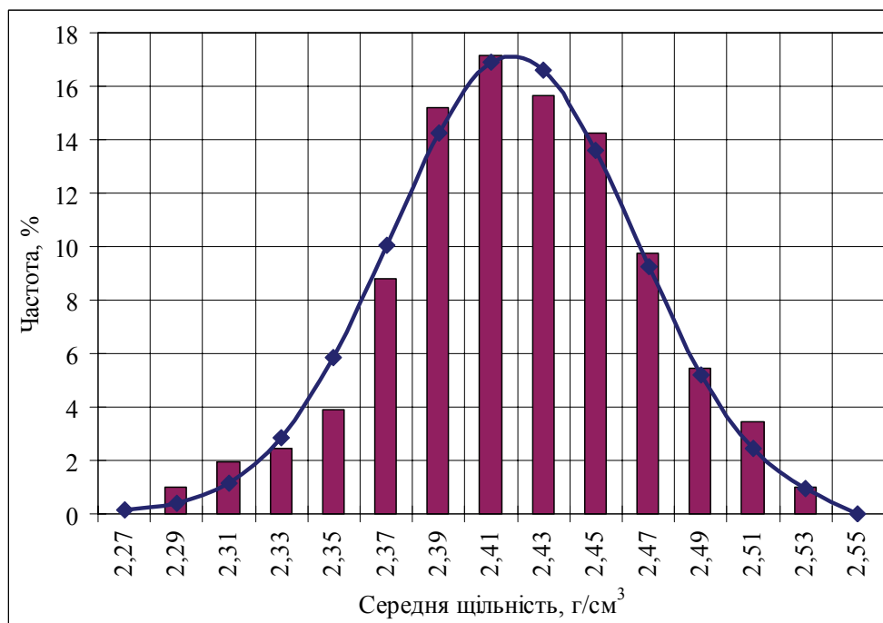
Рисунок 5 – Гістограма та щільність розподілу середньої густини цементобетонних зразків
