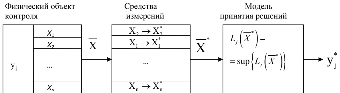
Рисунок. 2 – Структурная схема обработки результатов однократных измерений на этапе измерительного контроля
