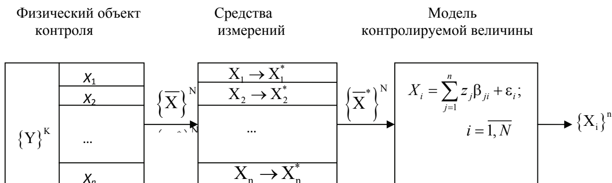
Рисунок 1 – Структурная схема процесса обработки результатов многократных измерений на этапе анализа обучающих выборок
