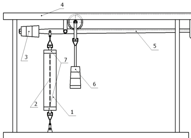
1 – зразок з армованого асфальтобетону; 2 – армуючий матеріал; 3 – вантаж для рівноваги консолі; 4 – станина (корпус); 5 – консоль; 6 – рухомий вантаж; 7 – металеві накладки
