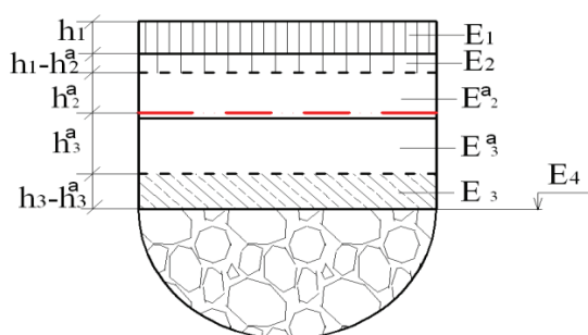
2а – конструкція з армованими асфальтобетонними шарами, як багатошарова конструкція з врахуванням впливу армування на розрахункові характеристики асфальтобетону
