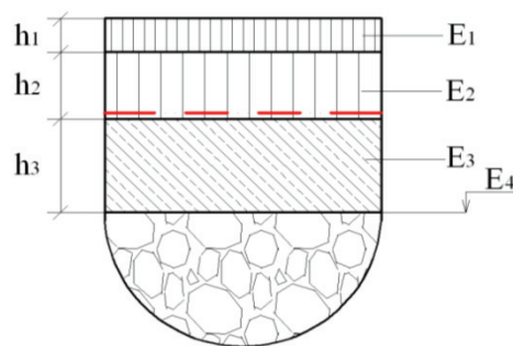
1 б – конструкція з армованими асфальтобетонними шарами
