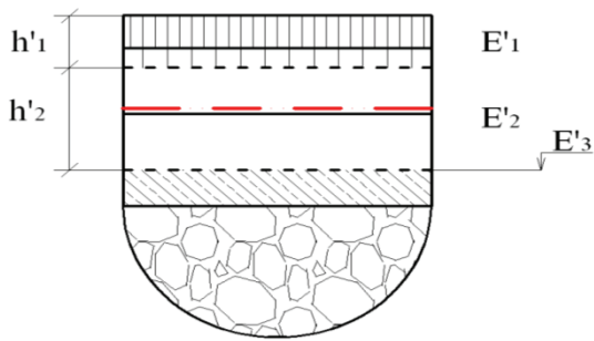
2б – конструкція з армованими асфальтобетонними шарами, приведена до тришарового напівпростору
