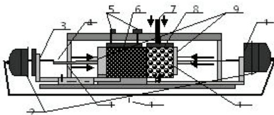
3а - схема випробування на зсув
